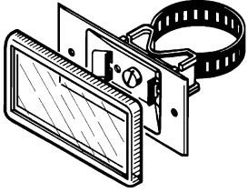
UNI univerzális tartó feszítőszalaggal
